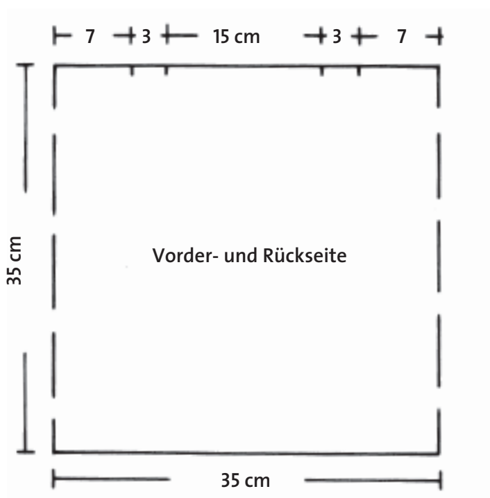
Schnittschema Tasche
